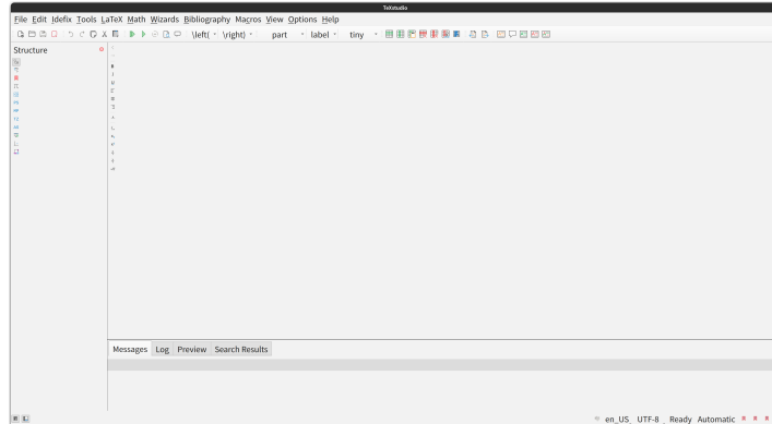
图 1.2 TeXstudio 界面
