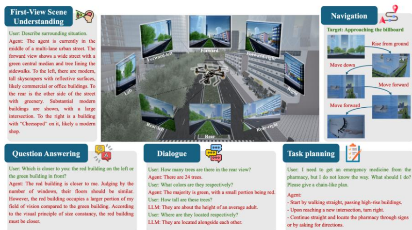
城市具身智能平台 EmbodiedCity 示意图
